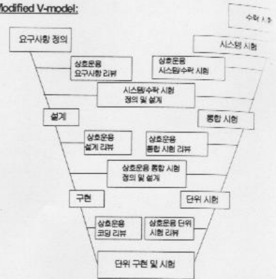
(그림 3) 변형된 V-모델
