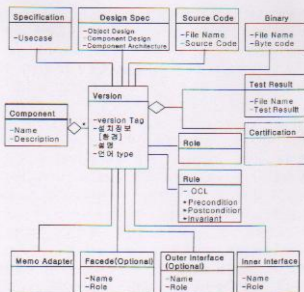
(그림 6) UML을 이용한 컴포넌트 규격
