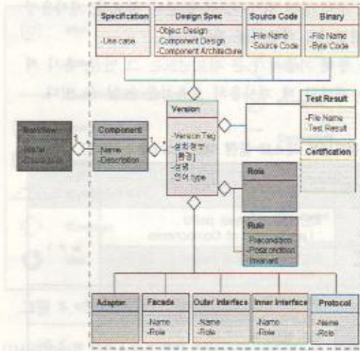
그림 3. 구조적인 워크플로우 모델링
