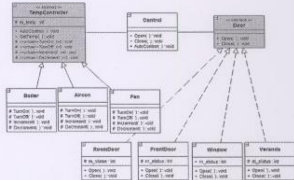
그림 7. 온도조절하기의 클래스 다이어그램 Fig. 7. Class Diagram of temperature control
