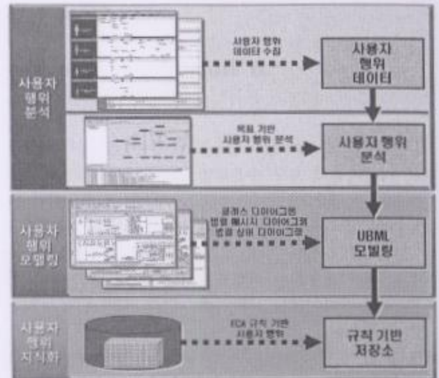
그림 1. 사용자 행위 분석 프레임워크 Fig.1. User Behavior Analysis Framework
