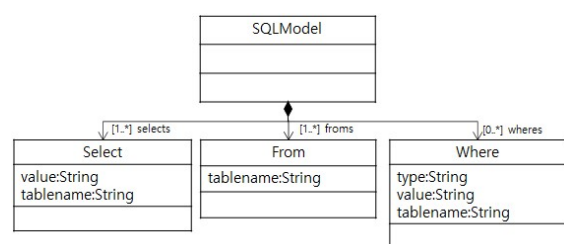
Fig. 5. SQL Metamodel
